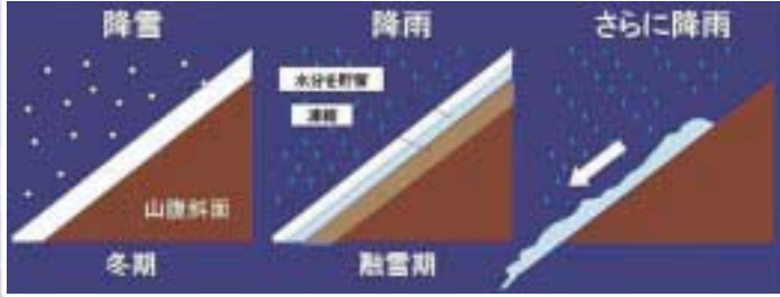
スラッシュ雪崩のメカニズム
